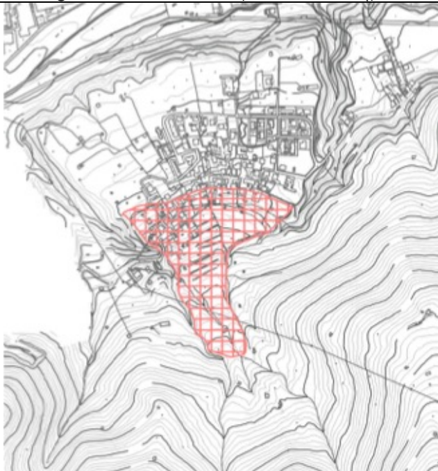
Conoide Stabello (Cn)
