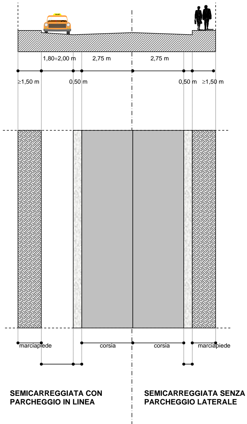
figura 3: SEZIONE TIPO STRADA LOCALE (a doppio senso di marcia)
