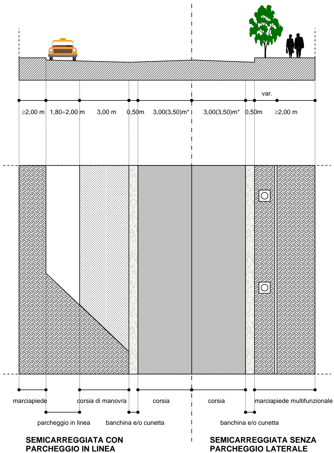
figura 1: SEZIONE TIPO STRADA DI QUARTIERE
