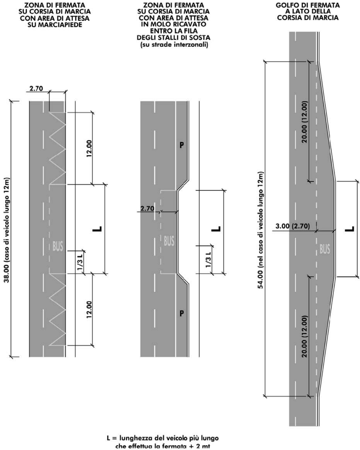
figura 5 - Zone e golfi di fermata dei mezzi pubblici collettivi
