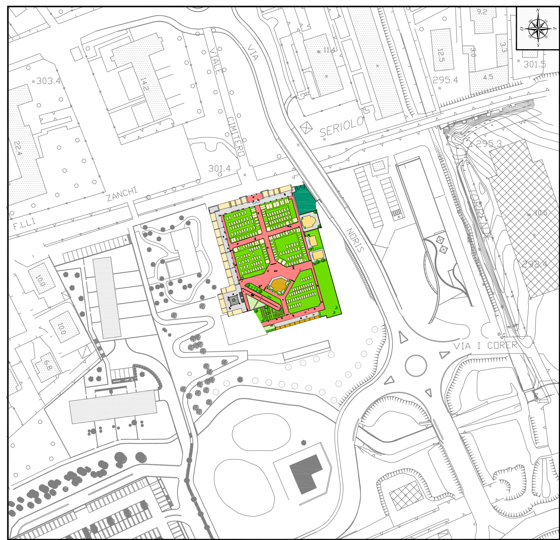
Inquadratura aerofotogrammetrica - scala 1:1.000
