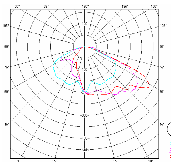
Figura 5.15 - Curva fotometrica di apparecchio asimmetrico misurata su 3 piani.
