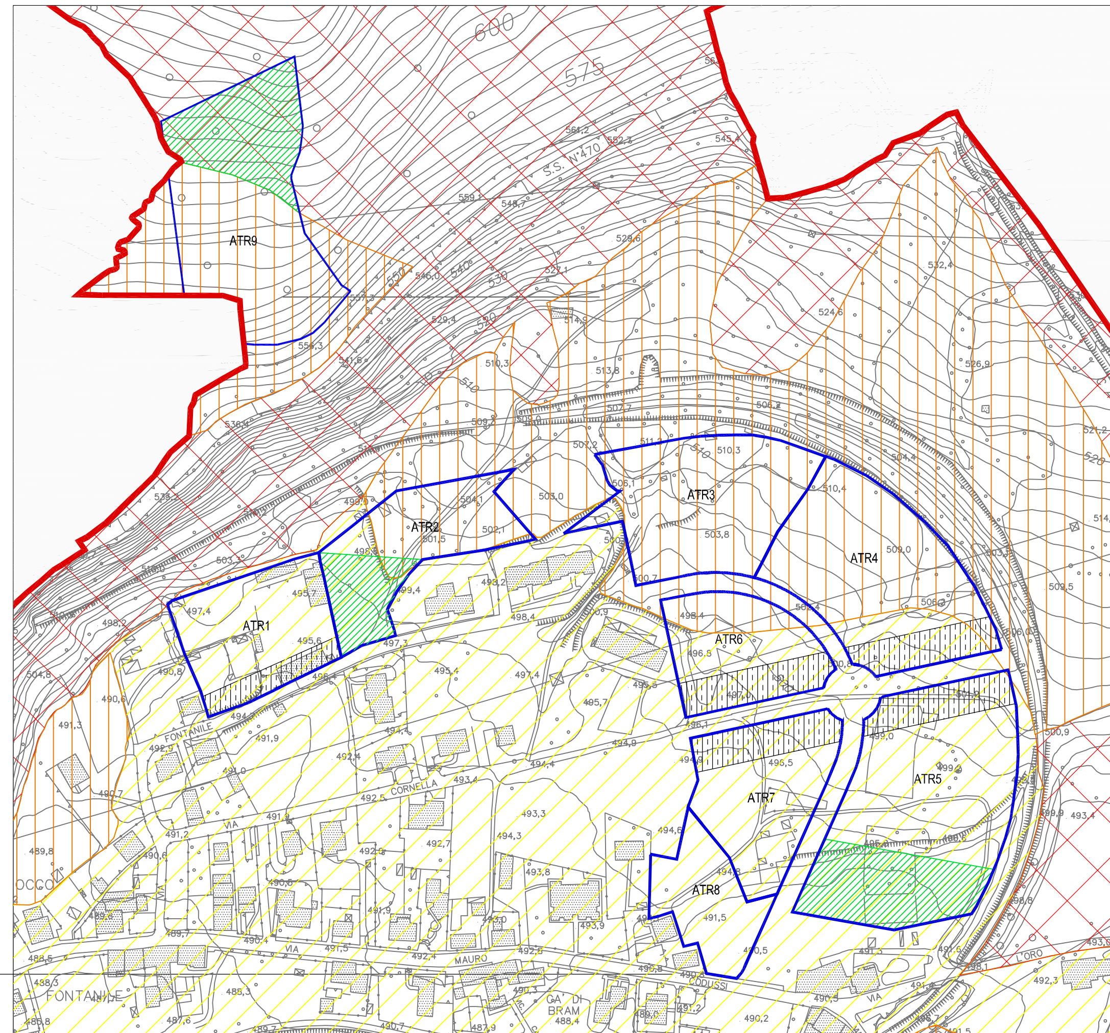
SOVRAPPOSIZIONE DELLE AREE DI TRASFORMAZIONE ALLA CARTA DI FATTIBILITA' GEOLOGICA
