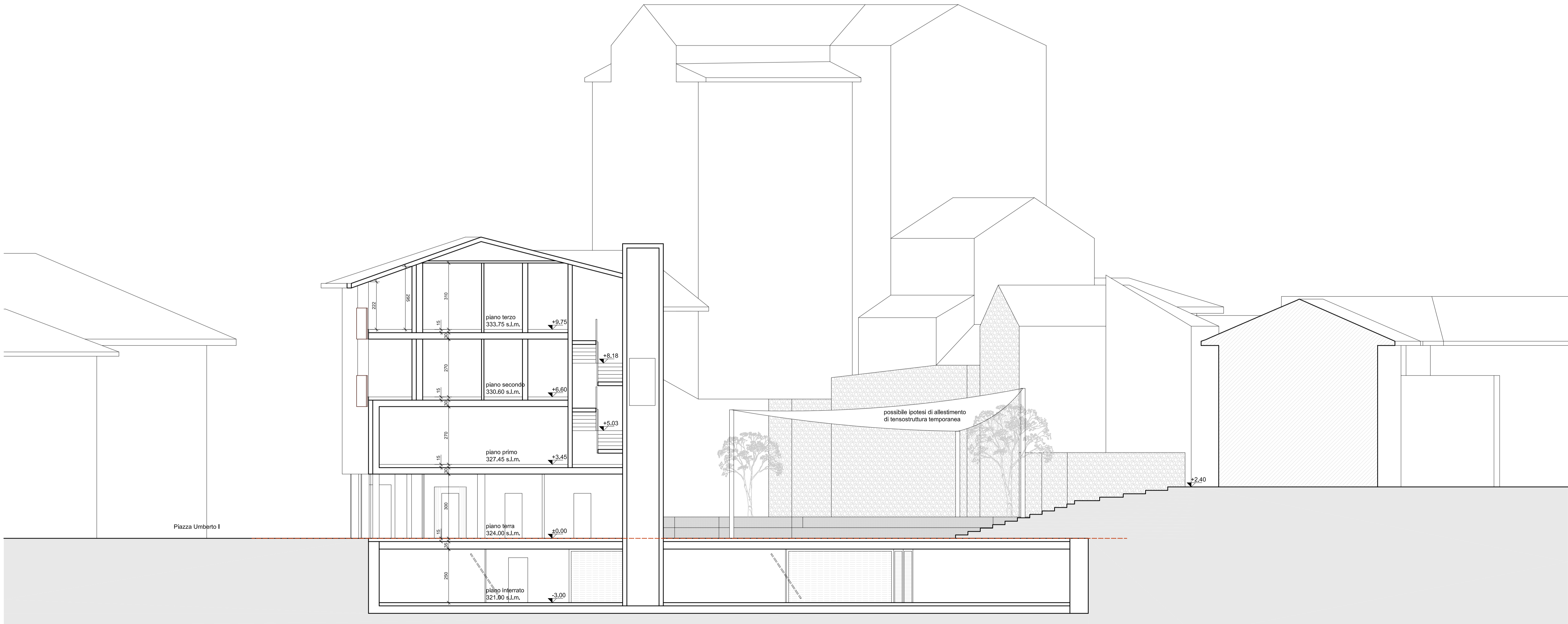
Sezione BB
