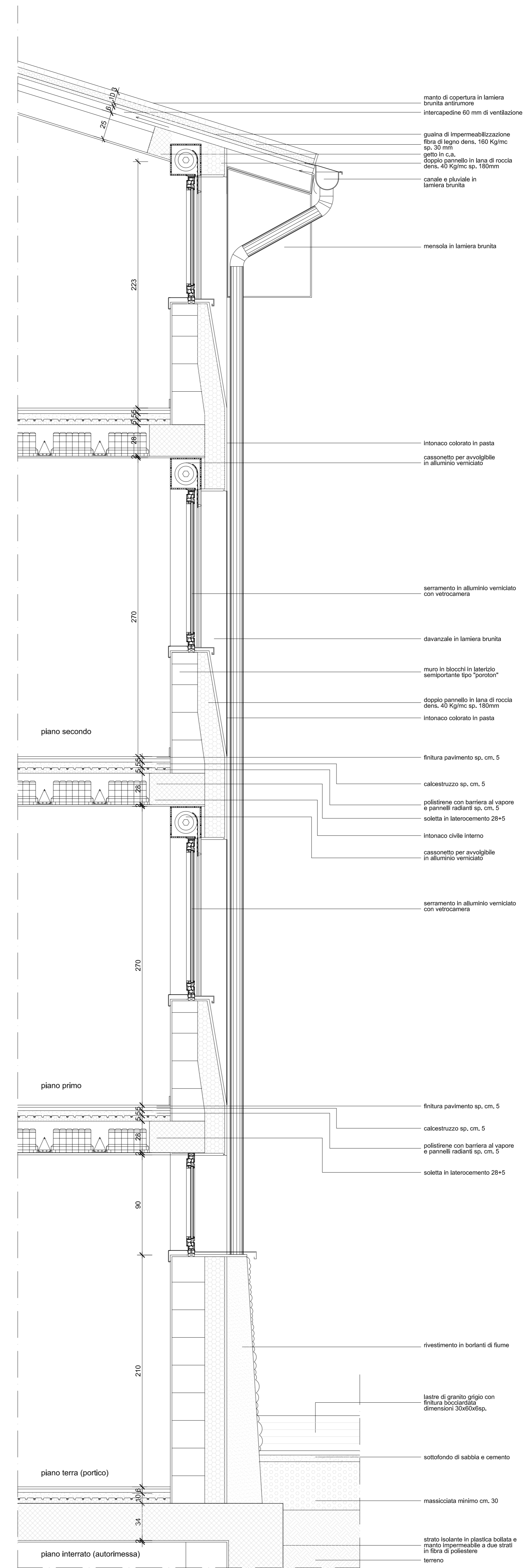
PORTICO E FACCIATA LATO VIA VITTORIA: sezione e prospetto
