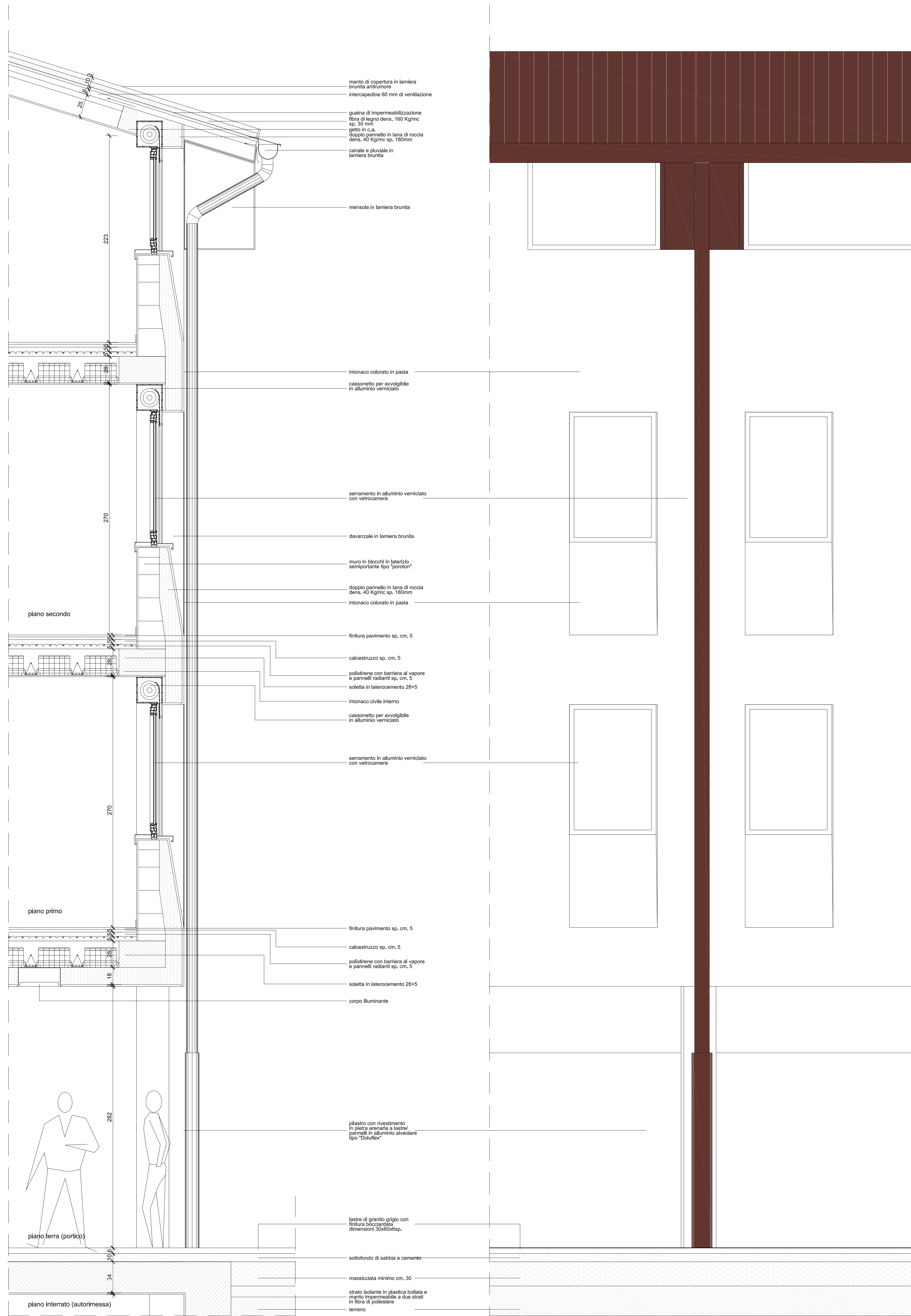
PORTICO E FACCIATA LATO PIAZZA UMBERTO I: sezione e prospetto
