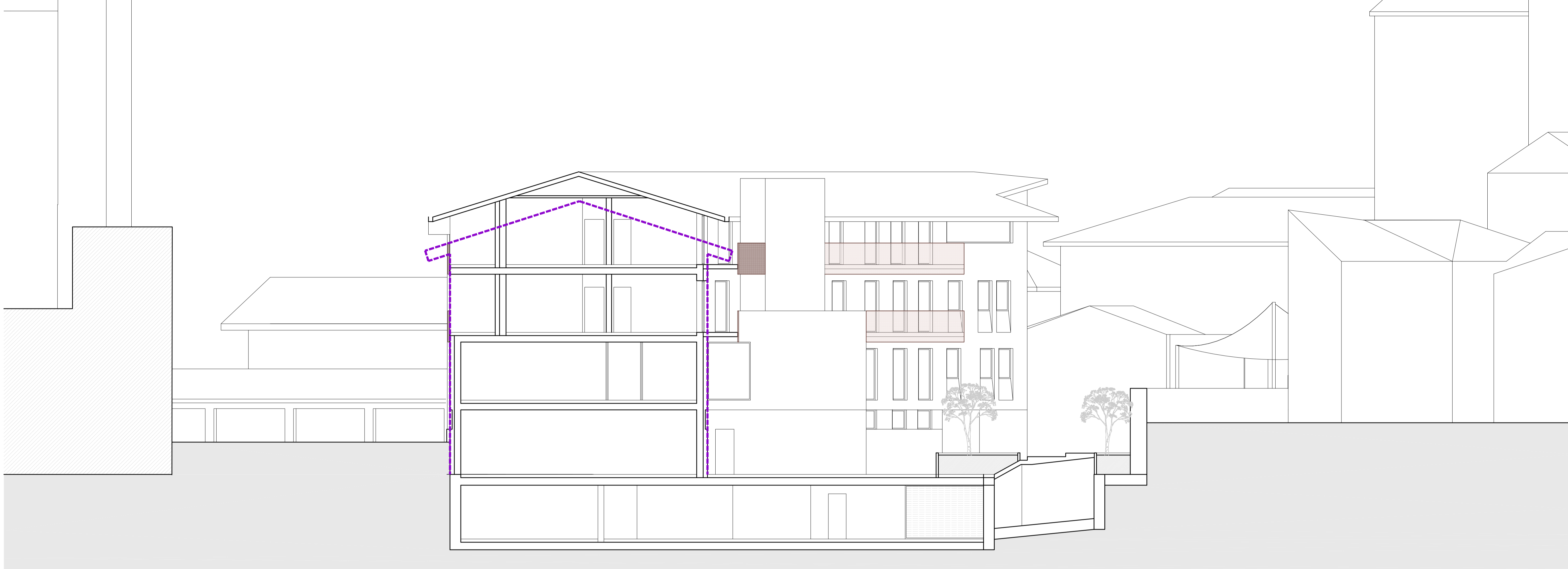
Sezione AA
