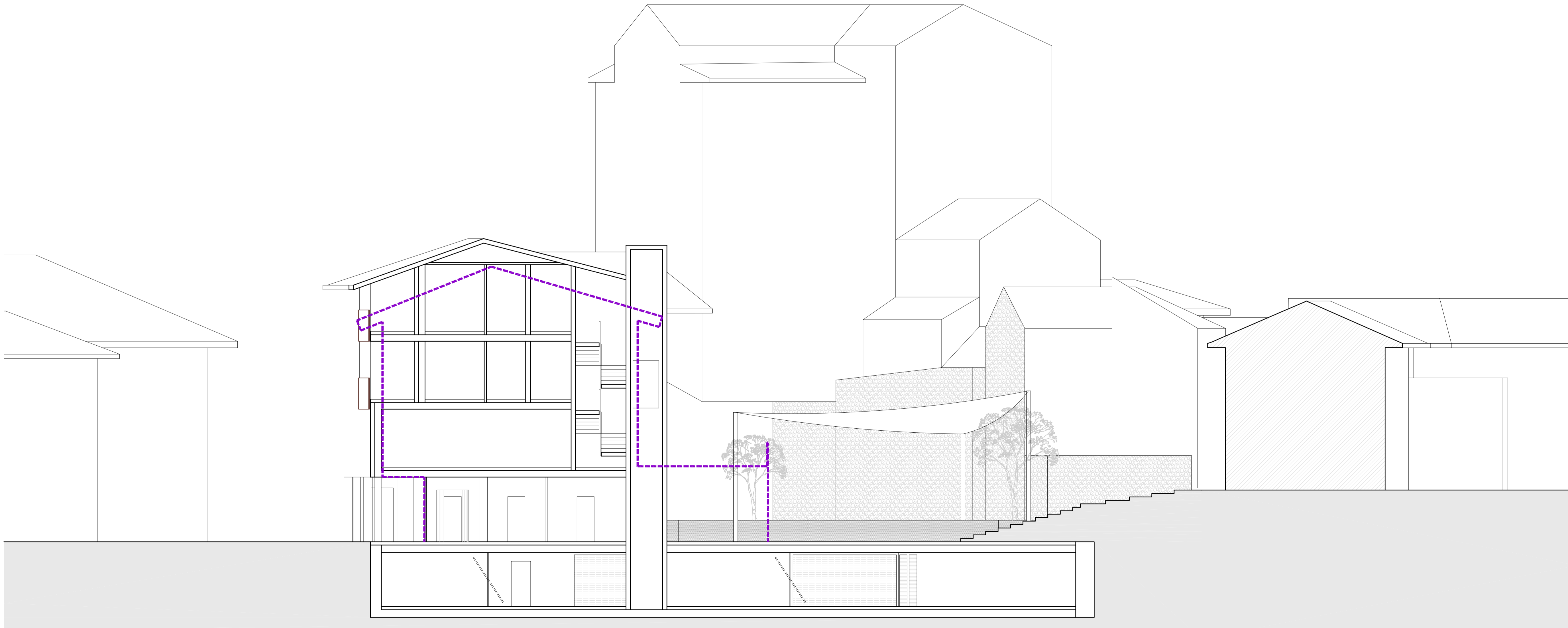
Sezione BB
