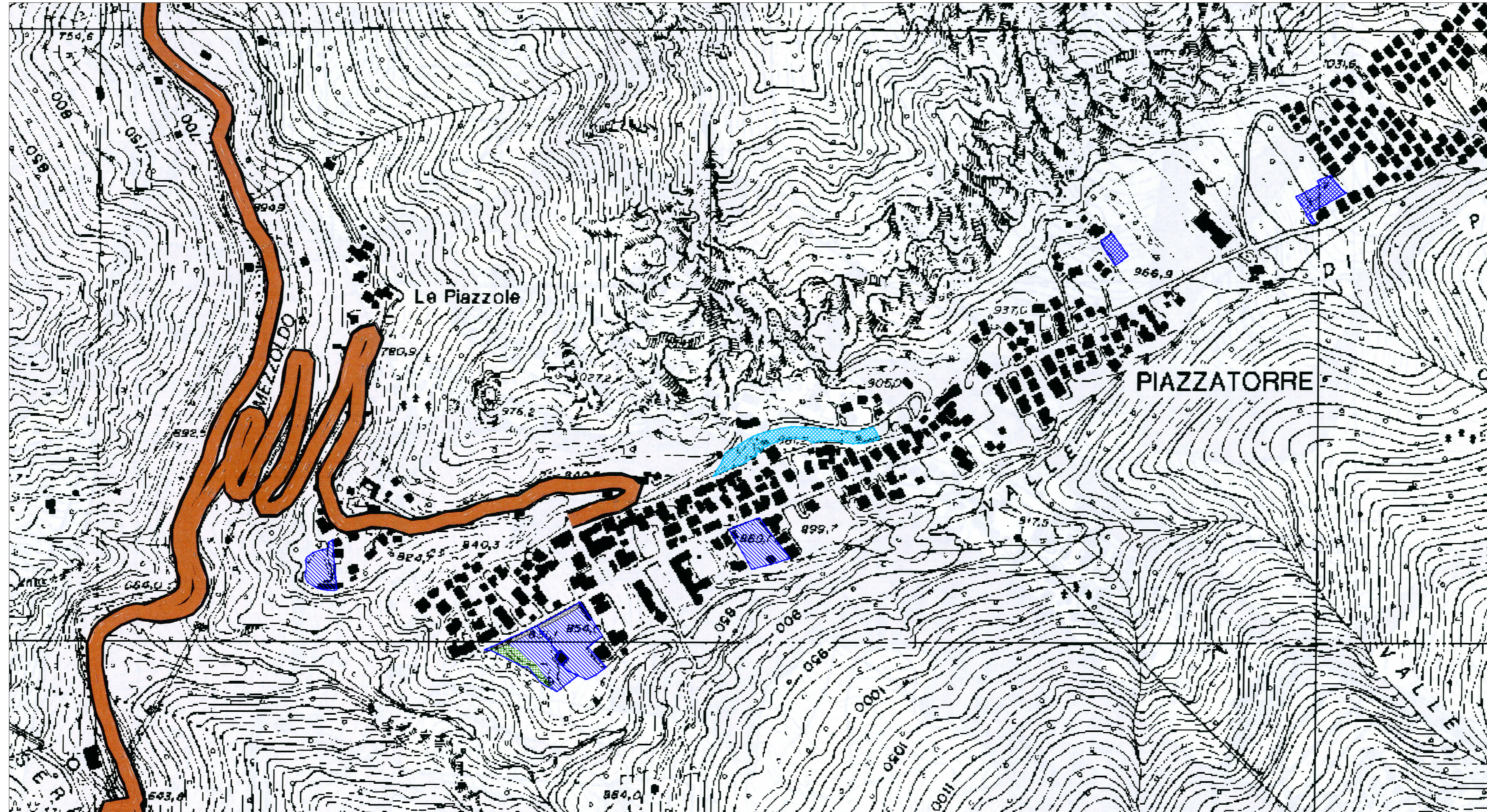
ESTRATTO CARTA E.3 DEL PTCP - INFRASTRUTTURE PER LA MOBILITA' scala 1:5.000
