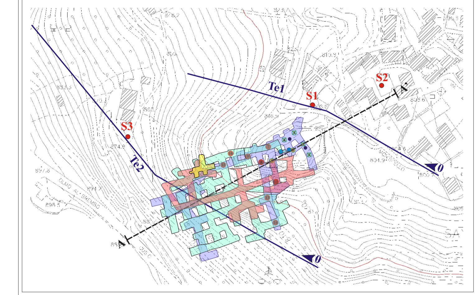
UBICAZIONE SEZIONE GEOLOGICA SCALA 1:2.000
